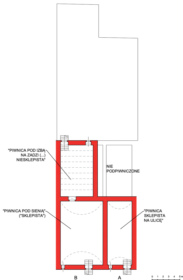
Il.2. Rzut piwnic kamienicy ul. Szewska nr 23.
